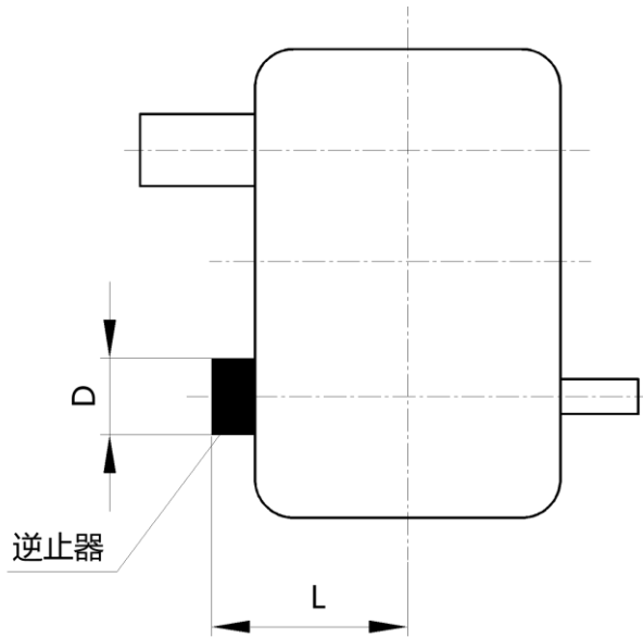
逆止器安装尺寸
